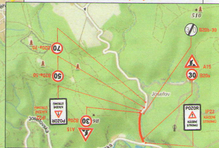
označení pracovního místa v době umožnění průjezdu
